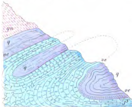
Fig. 3. Profil durch die Faltungen am Jäggigrätli (Mettenberg).
